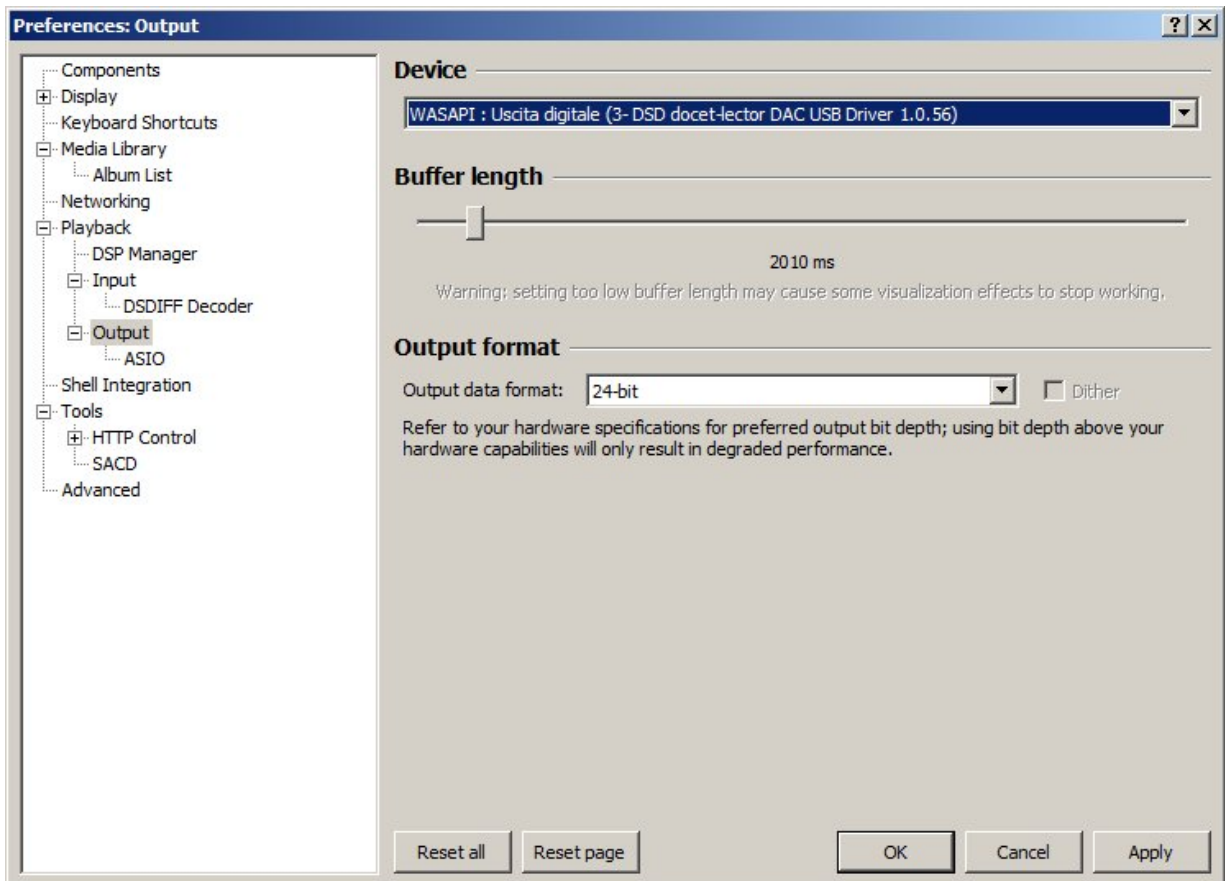
Bedienfeld „Ausgabeeinstellungen“ mit Wasapi-Treiber
